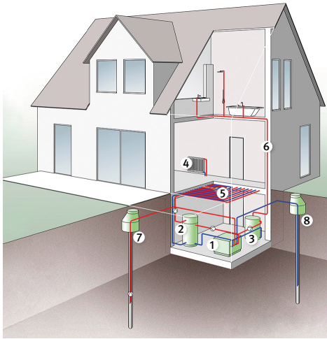
1 Wärmepumpe 2 Pufferspeicher 3 Trinkwarmwasserspeicher 4 Radiator 5 Flächenheizung 6 Warmwasserleitung 7 Entnahmehauptbrunnen mit Brunnenkopf 8 Schluckbrunnen mit Brunnenkopf
